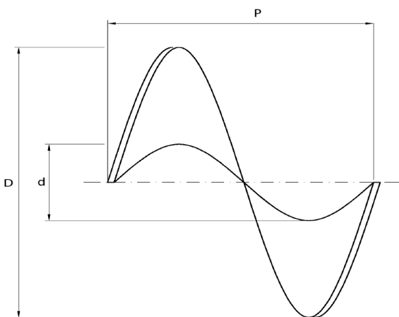
Plano de un sinfín espira.
